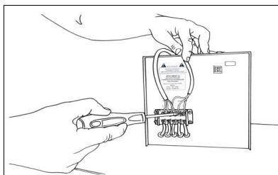
Рис. 8. Подключение стабилизатора через клеммную колодку
